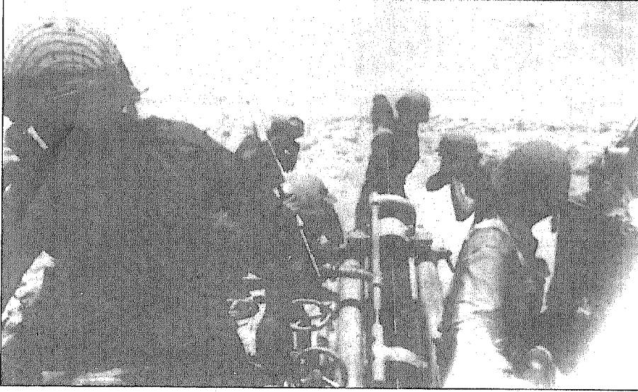
هاون من عيار ١٦٠ مم (سلطان) أثناء تجميعه. استخدمته معظم الوحدات الميكانيكية الإسرائيلية بدلا من المدفعية، ويمكن تحميله في العربات المجنزرة.
