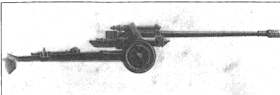
مدفـع ميدان عيار ۱۳۰ مم.
