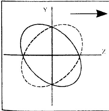
E- الحالة الأولى لاستقطاب الموجة التجاذبية الصرف
