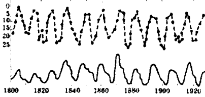
تأثير كواكب المشتري والأرض والزهرة وعطارد على نشاط الشمس - الخط البياني العلوي: توزيع الكواكب - الخط البياني السفلي: نشاط الشمس
